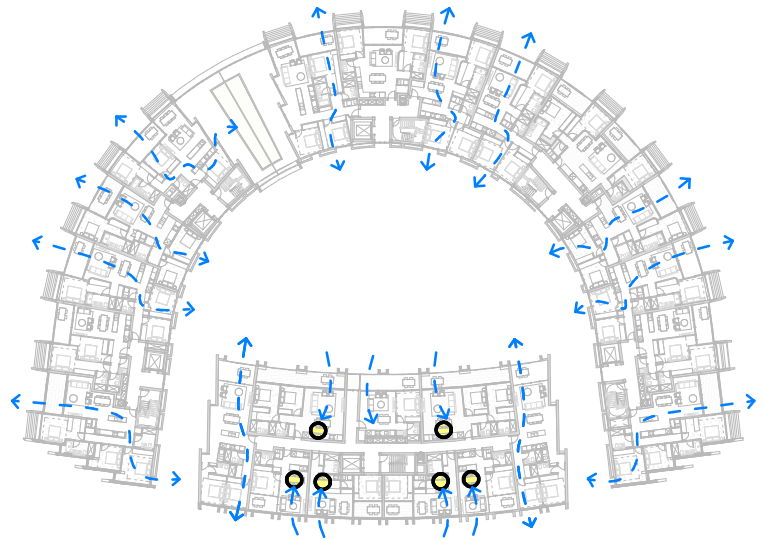
4 CROSS-VENTILATION - L03 1 : 500
