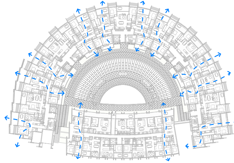
2 CROSS-VENTILATION - L01 1 : 500
